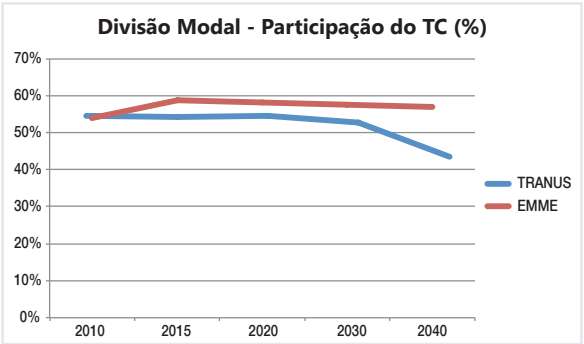
Figura 4.2 Divisão Modal dos dois softwares na hora pico
