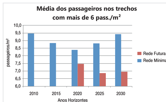
Figura 4.25 Média dos passageiros nos trechos com mais de 6 pass./m 2 – EMME
