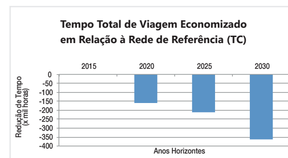
Figura 4.6 Tempo total economizado nas viagens por TC (hora pico da manhã) – EMME
