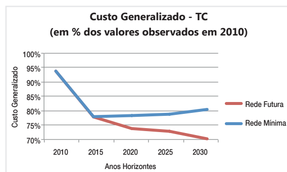
Figura 4.4 Custo Generalizado TC na hora pico da manhã – EMME
