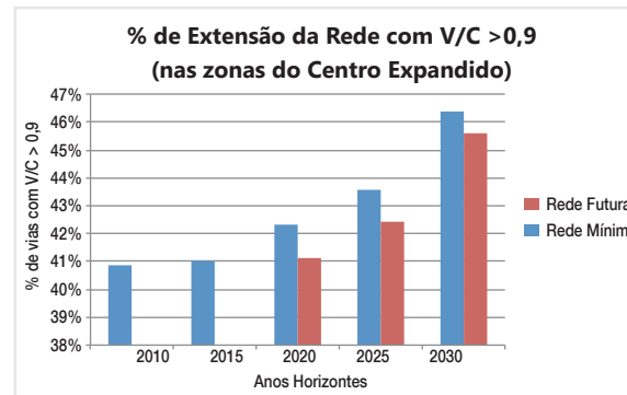
Figura 4.7 Taxa de Saturação Viária nas zonas de tráfego do Centro Expandido (hora pico da manhã) – TRANUS
