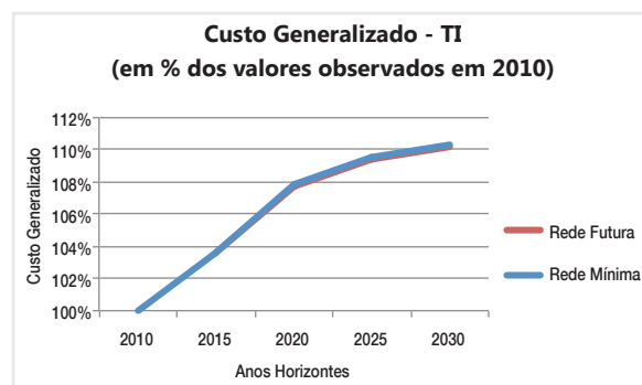
Figura 4.3 Custo Generalizado do TI na hora pico da manhã – EMME
