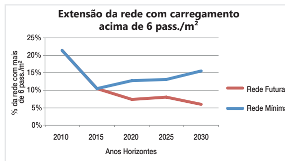
Figura 4.24 Extensão da Rede com carregamento acima de 6 passageiros/m 2 – EMME
