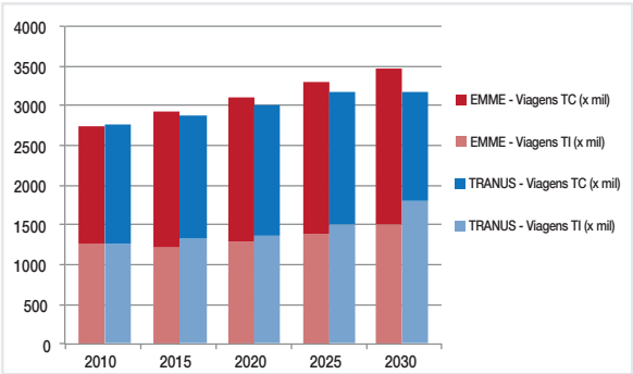
Figura 4.1 Totais de viagens dos dois softwares na hora pico
