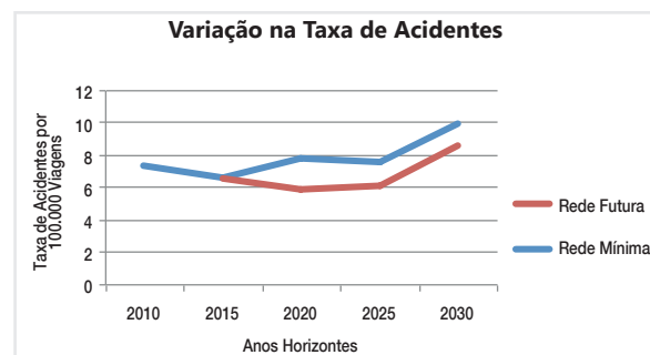
Figura 4.12 Taxa de Acidentes por 100.000 viagens – TRANUS
